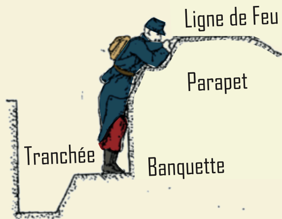
Aménagement individuel d'une tranchée.
